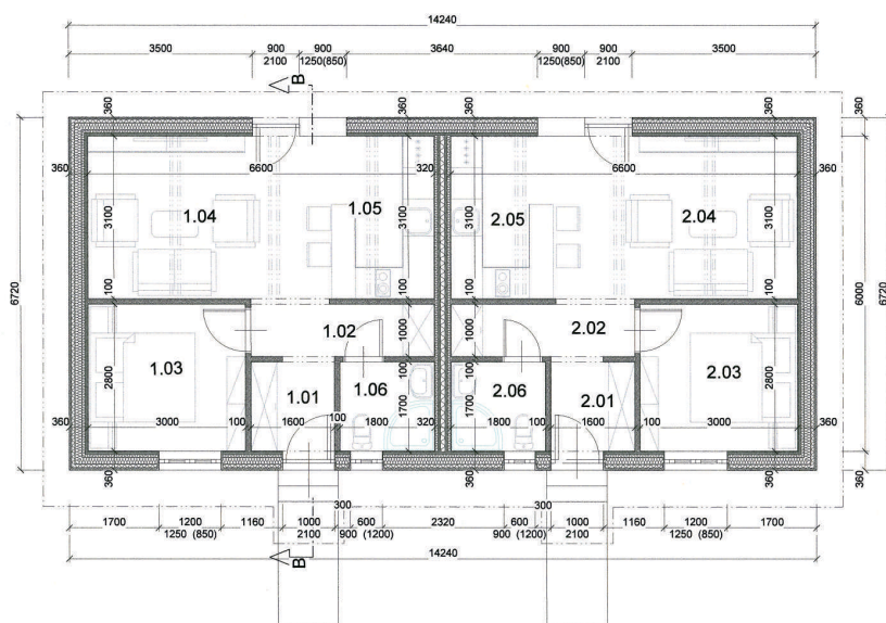
LEGENDA MÍSTNOSTÍ: BEZ ÚLOŽNÉHO PROSTORU V 1NP
