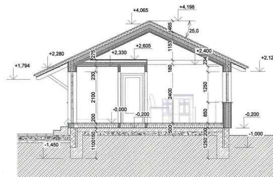
VZOROVÝ PŘÍČNÝ ŘEZ
